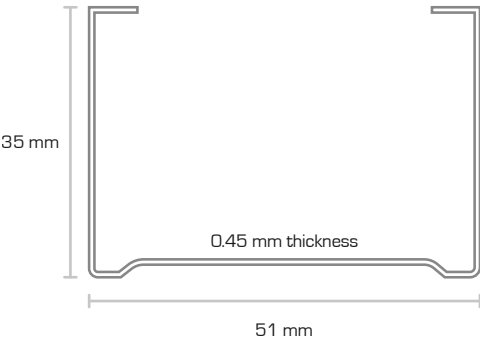
Stud 51x35x0.45
