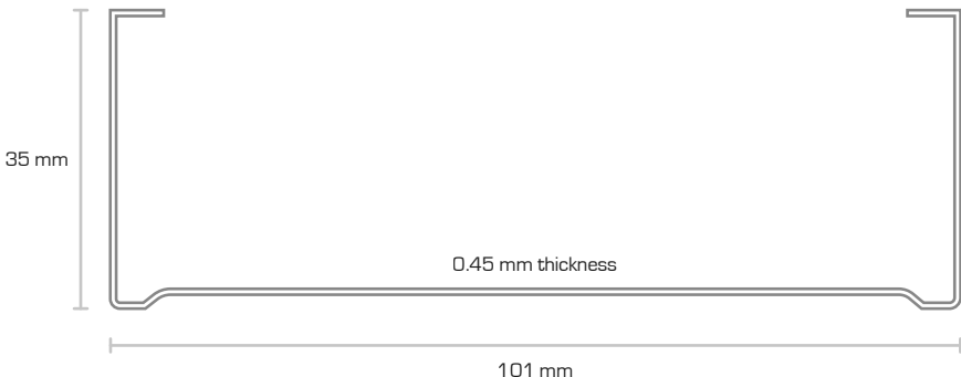
Stud 101x35x0.45
