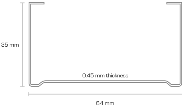
Stud 64x35x0.45
