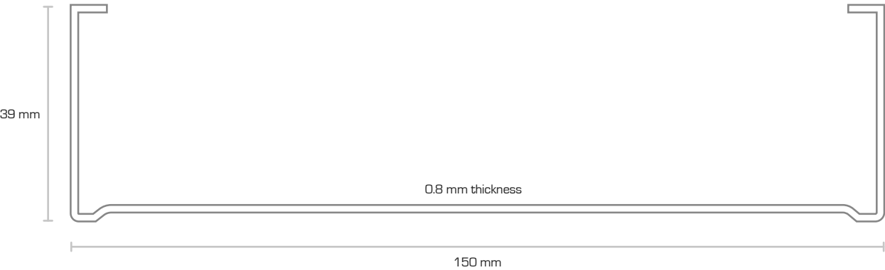
Stud 150x39x0.8
